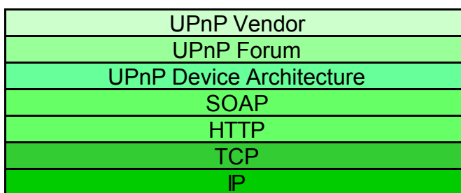
Figura 14: Livelli dello stack UPnP utilizzati da un messaggio di tipo control
