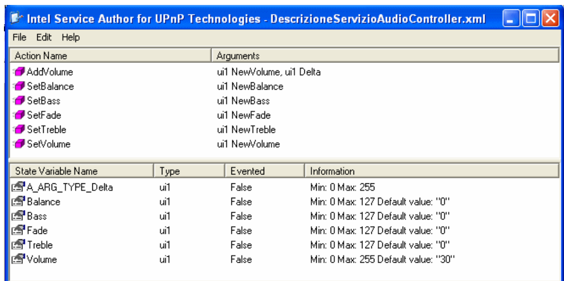
Figura 27: Schermata della finestra del tool Intel Service Author dopo la definizione delle Variabili di Stato e delle Azioni del servizio.
