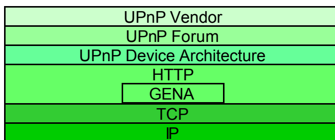
Figura 15: Livelli dello stack UPnP utilizzati da un messaggio di tipo event e subscription
