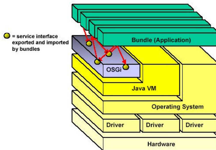
Figura 6: Ambiente OSGI
