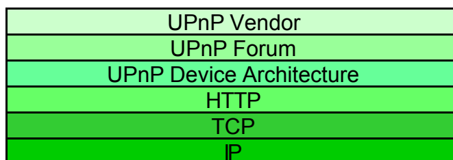
Figura 18: Livelli dello stack UPnP utilizzati per recuperare una pagina di presentazione.
