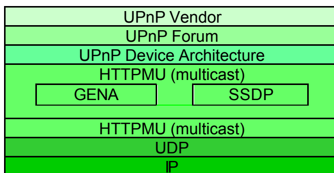
Figura 8: Livelli dello stack UPnP utilizzati da un messaggio di advertising della fase discovery
