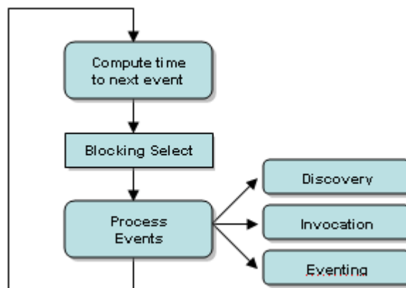
Figura 26: Schema di esecuzione di un thread
